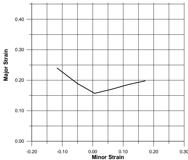
الشكل (11) منحنى حد التشكيل لصفحة من سبيكة الألمنيوم (2024-T3) كما مستلمة (As Recieved)
